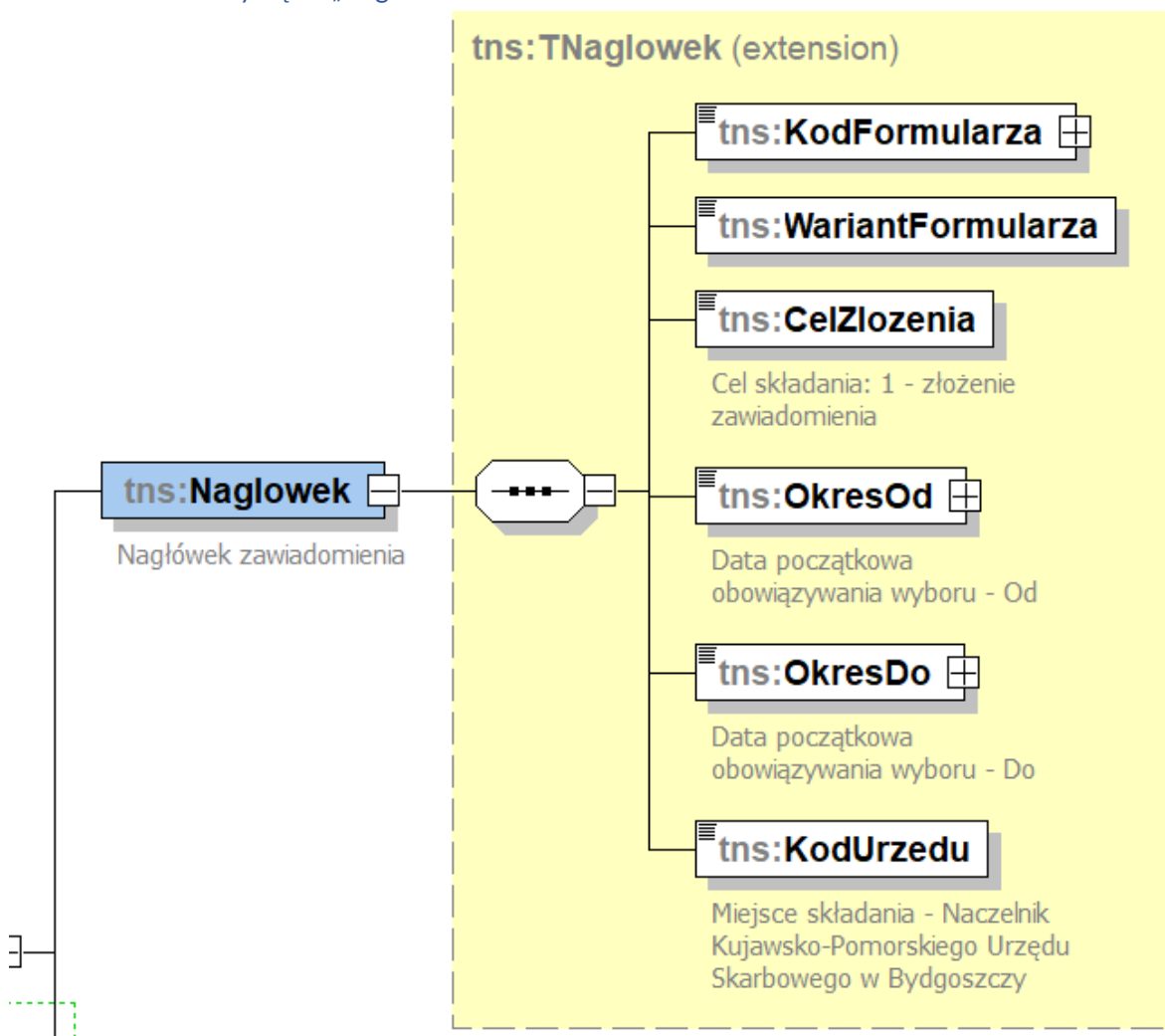
Schemat. 2 Struktury węzła „Naglowek” zawiadomienia GLB-Z3
