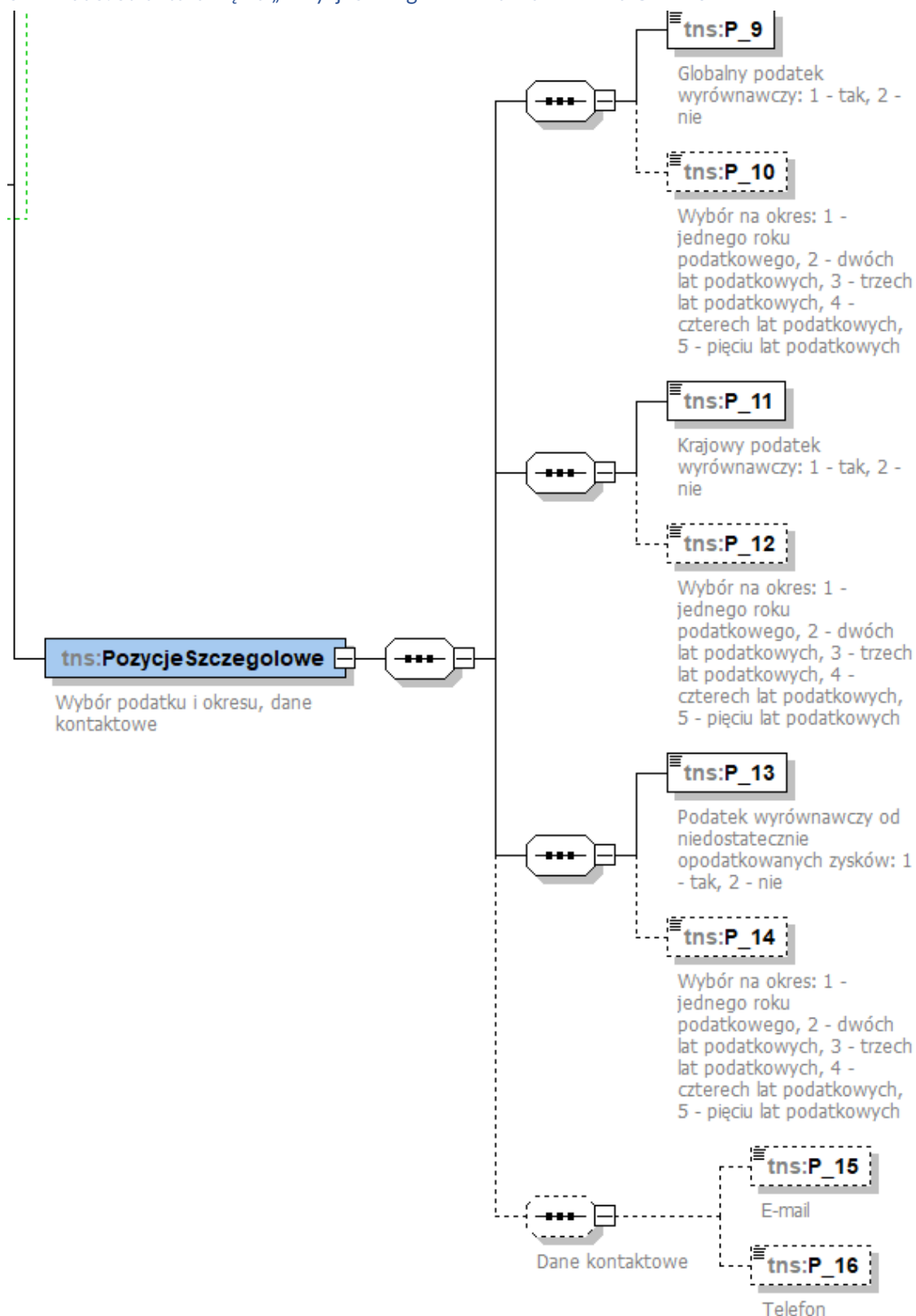
Schemat 5. Struktura węzła „PozycjeSzczegolowe” zawiadomienia GLB-Z3
