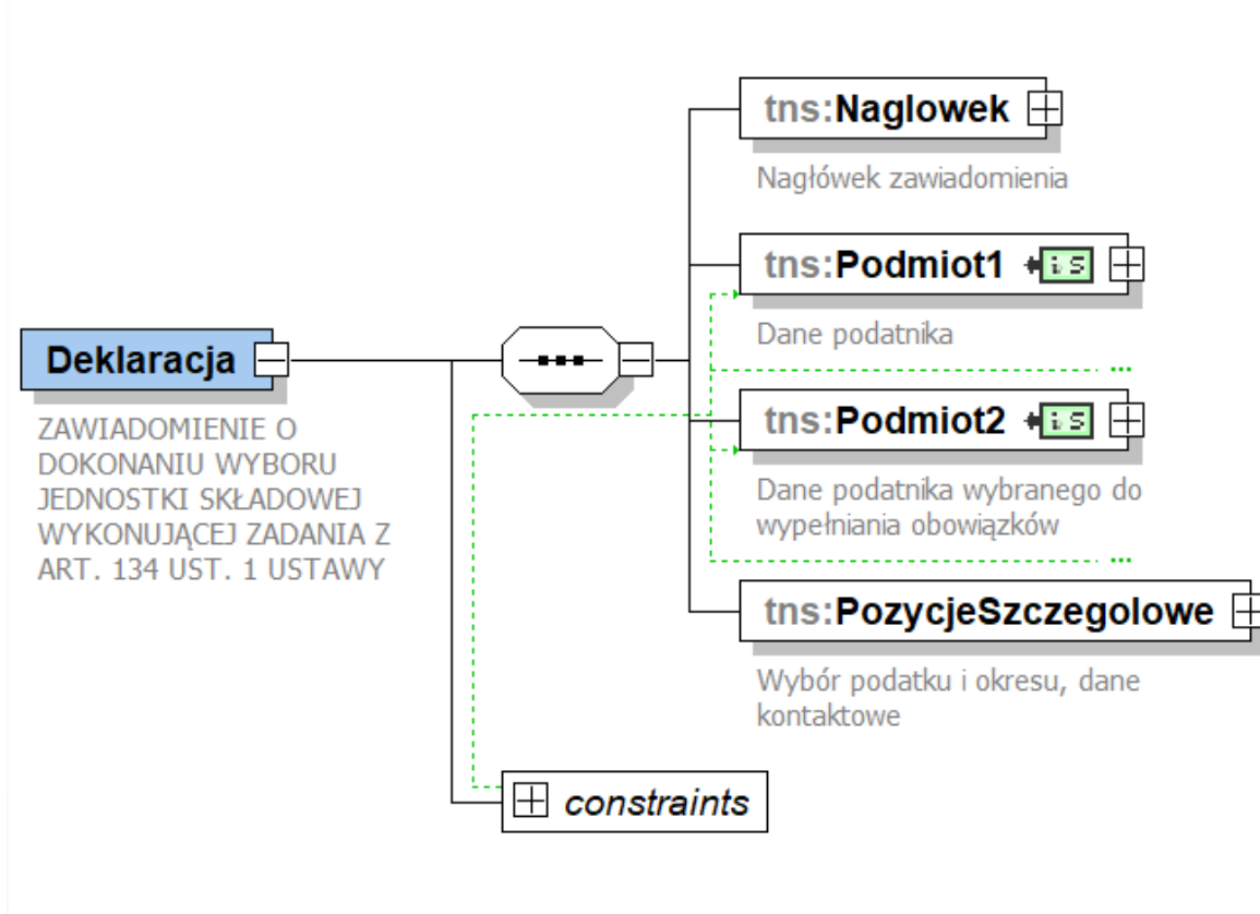
Schemat 1. Struktura zawiadomienia GLB-Z3
