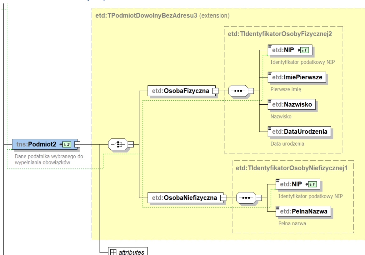
Schemat 4. Struktura węzła „Podmiot2” zawiadomienia GLB-Z3
