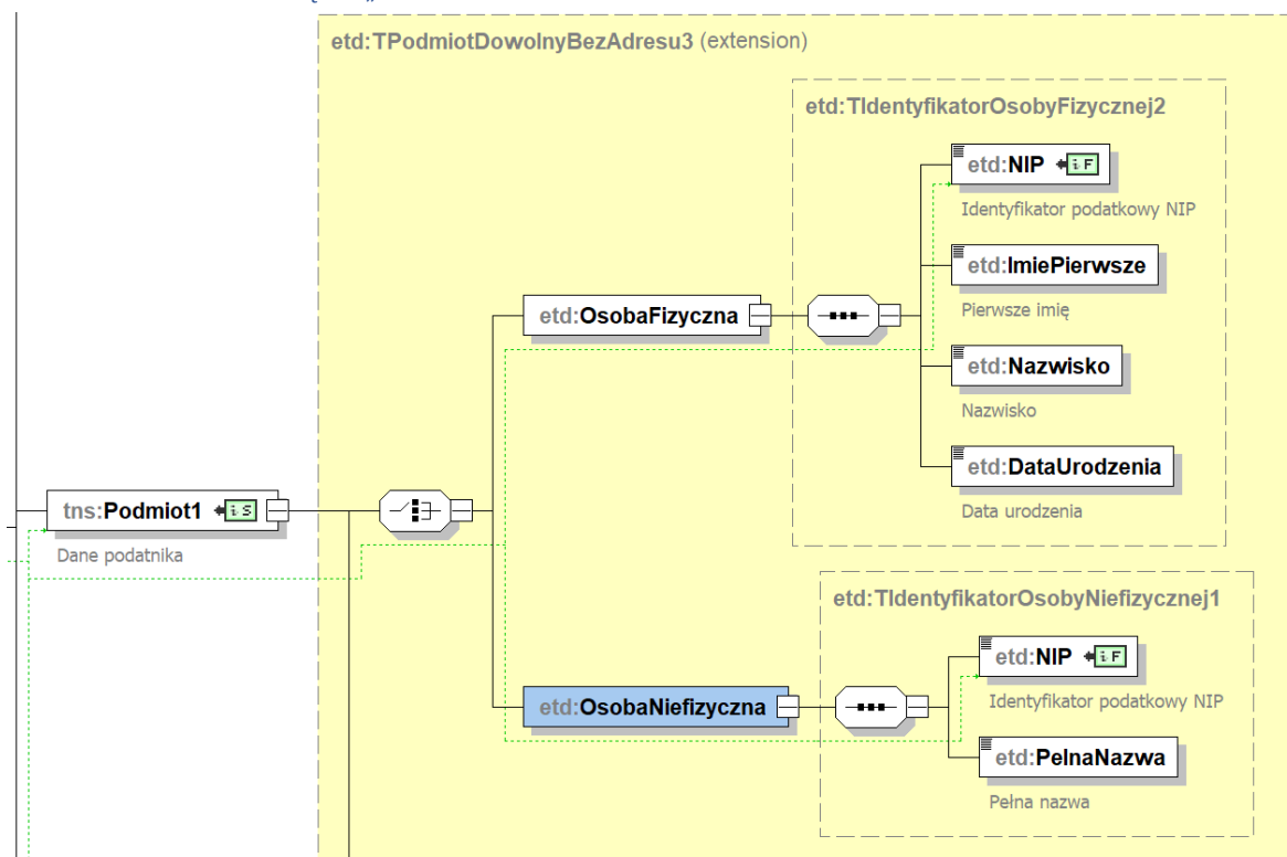
Schemat 3. Struktura węzła „Podmiot1” zawiadomienia GLB-Z3
